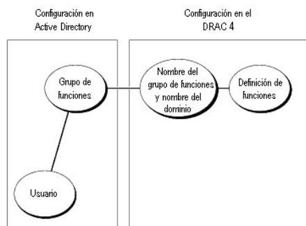
Figura 5-4. Configuración del DRAC 4 con Microsoft Active Directory y esquema estándar
