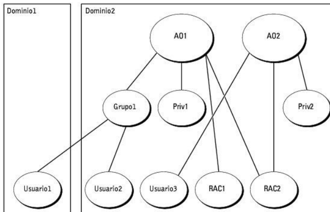
Figura 5-3. Configuración de los objetos de Active Directory en varios dominios
